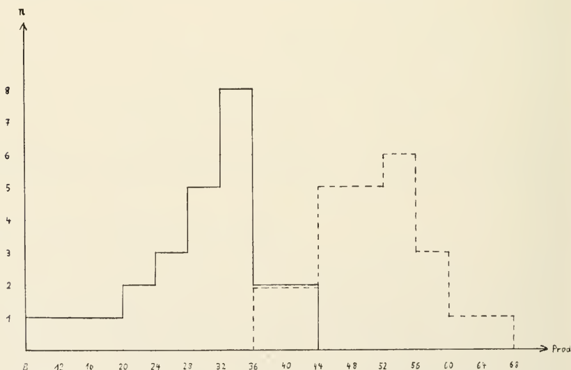
Abb. 4: Häufigkeitsverteilung der Produkte zweier Merkmale (Vorderflügelänge und Ozellendurchmesser) Klassenbreite d = 4 . Auffallend sind die deutliche Trennung der Maxima beider Subspezies und der geringe Transgressionsbereich.
